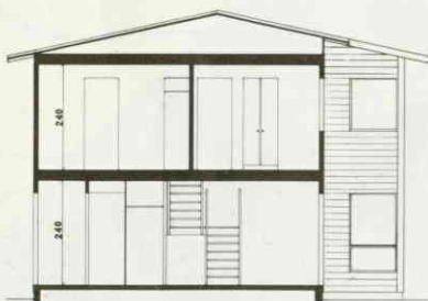
SNITT
